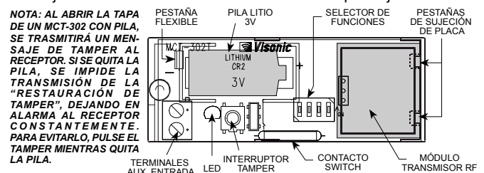
Figura 1. MCT-302 N con la tapa quitada
